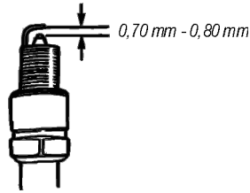
Fig. 25 – distancia de la bujía
