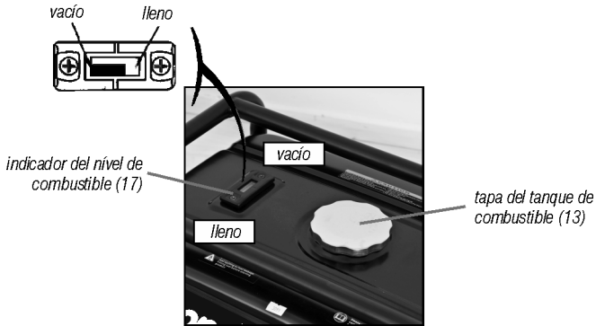
Fig. 8 – indicador del nivel de combustible
