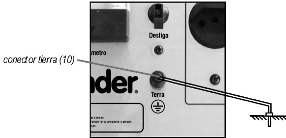
Fig. 14 – puesta a tierra del generador
