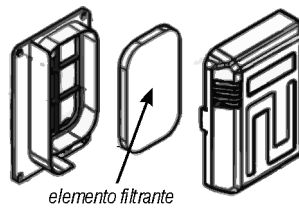
Fig. 21 – elemento filtrante
