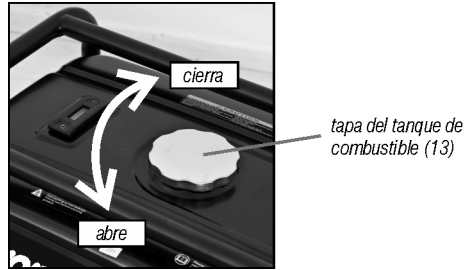
Fig. 9 – tapa del tanque
