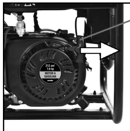
Fig. 18 – manija del sistema de arranque
