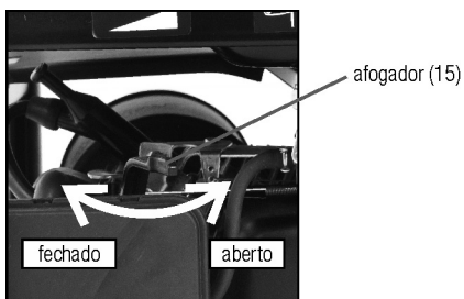
Fig. 12 – afogador
