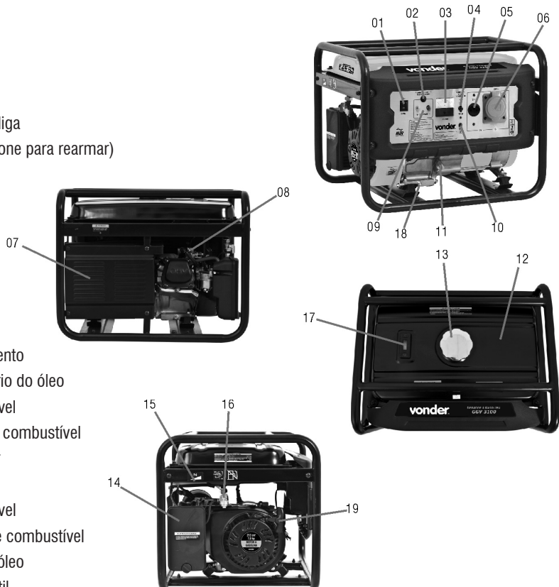
Fig. 5 – componentes
