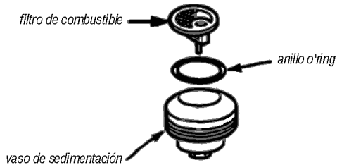
Fig. 23 – limpieza de los componentes
