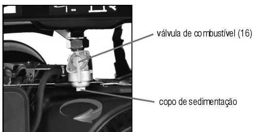
Fig. 22 – removendo copo de sedimentação
