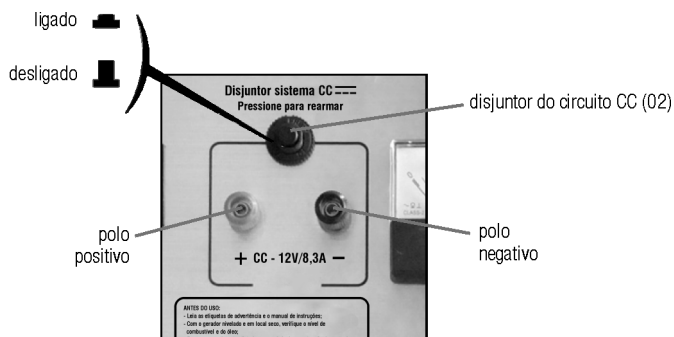
Fig. 16 – disjuntor do circuito CC
