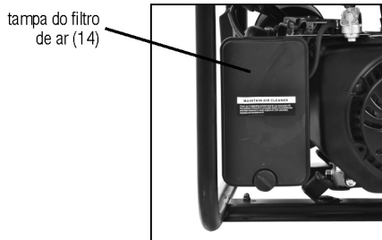
Fig. 20 – retirando a tampa do filtro de ar
