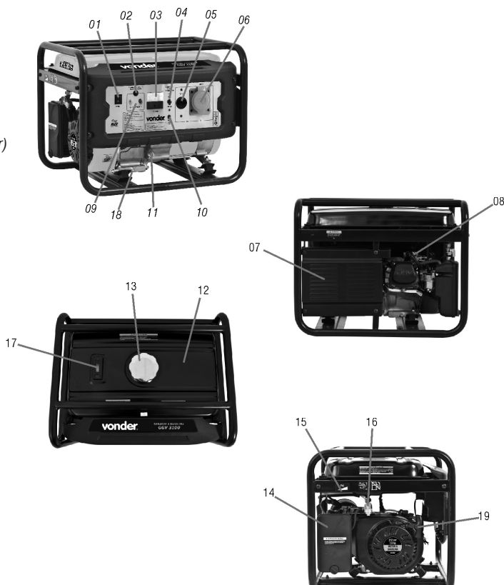
Fig. 5 – componentes
