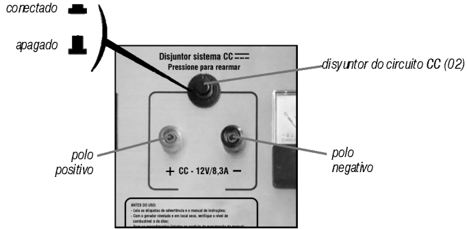
Fig. 16 – disyuntor del circuito CC
